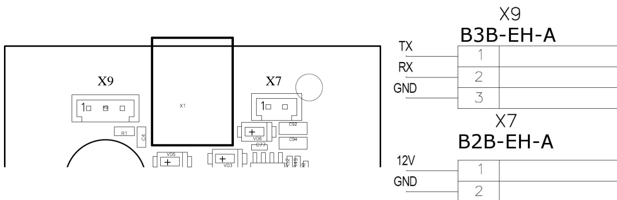
Рис.1 Подключение считывателя UEM NFC по интерфейсу RS232 и внешнему питанию.
